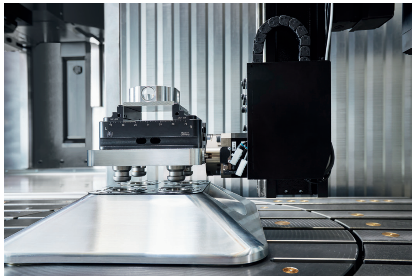
Basisvorrichtung für Automation auf dem Rundtisch. Spannung der Werkstückpaletten über Nullpunktspannsystem. Palettengrößen von 150 x 150 mm bis 800 x 800 mm.
