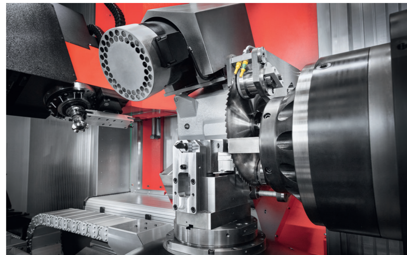
Übergabestation mit Spannstock auf Linearachse „U“ und Rundachse „C“, 2-Achs-CNC-Sägeeinheit.
