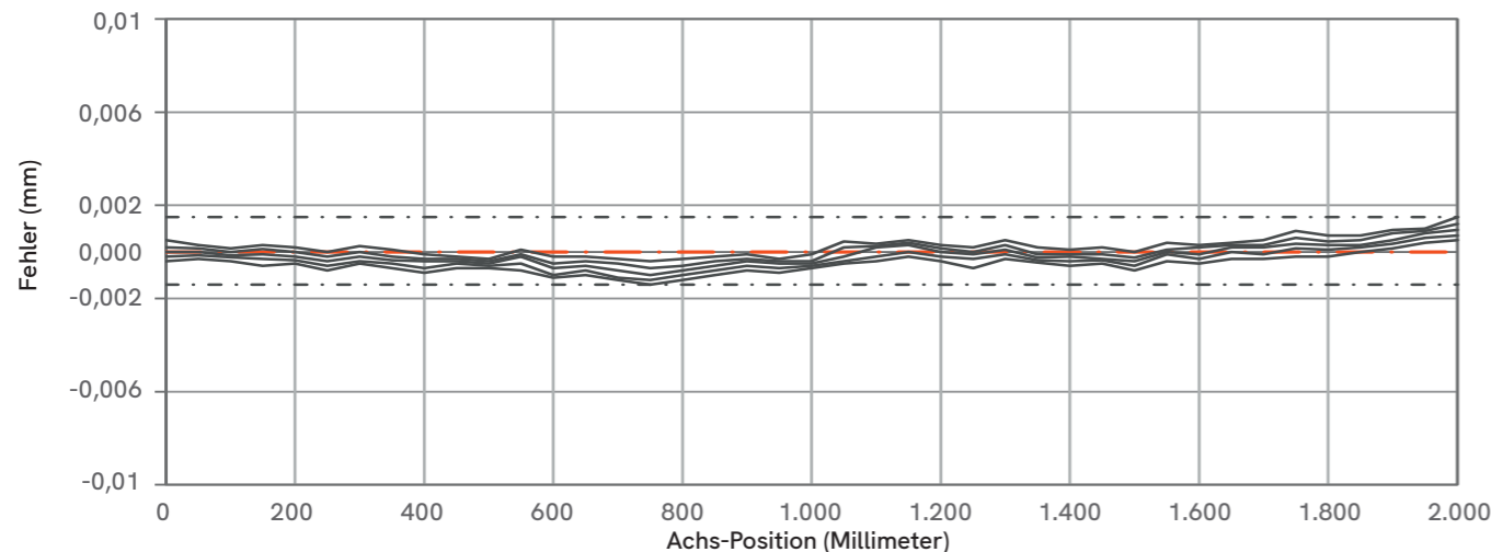
Norm: VDI/DGQ 3441 (Beispiel: Laservermessung Kugelrollspindel X-Achse) Positionsunsicherheit P gesamt 2,847 µm auf 2000 mm Achslänge
