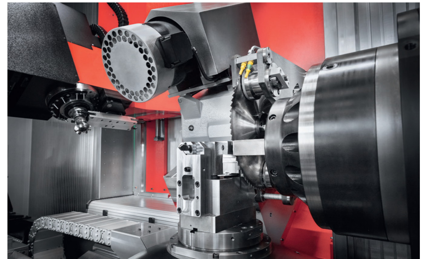
Übergabestation mit Spannstock auf Linearachse „U“ und Rundachse „C“, 2-Achs-CNC-Sägeeinheit.
