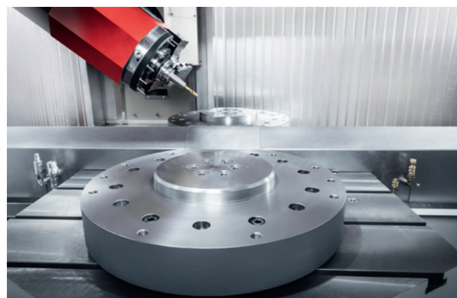
Abbildung der beiden Arbeitsräume mit geöffneter Sicherheitstrennwand.
