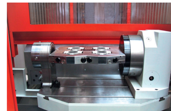
Arbeitsraum 1: Aufbau mit Rundtisch, Vorrichtungbrücke und Gegenlager. Mehrseitenbearbeitung.
