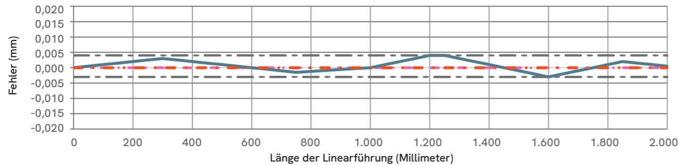
Norm: VDI/DGQ 3441 (Beispiel: Laservermessung Kugelrollspindel X-Achse) Positionsunsicherheit P gesamt 2,847 µm auf 2000 mm Achslänge
